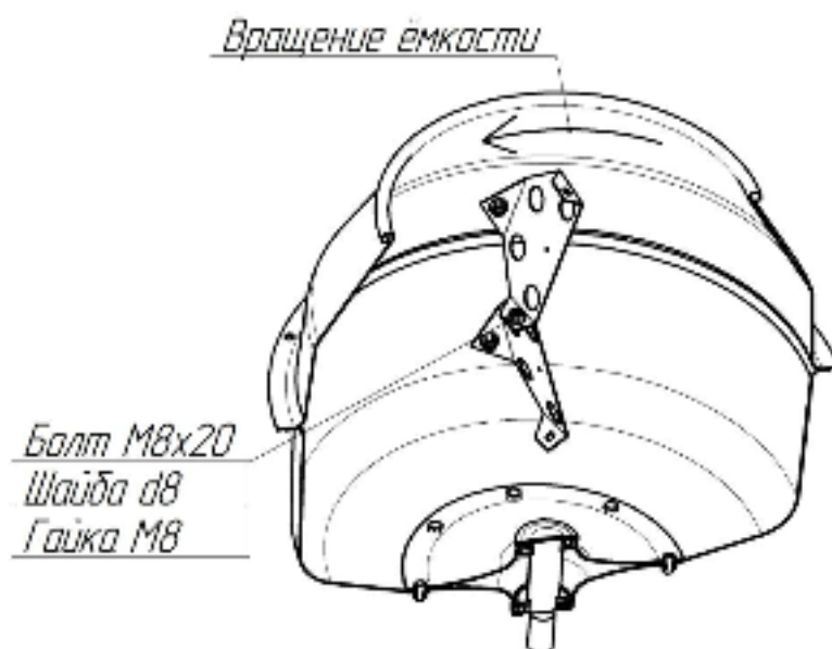
Рис. 2 Ёмкость со сборной лопастью в разрезе
